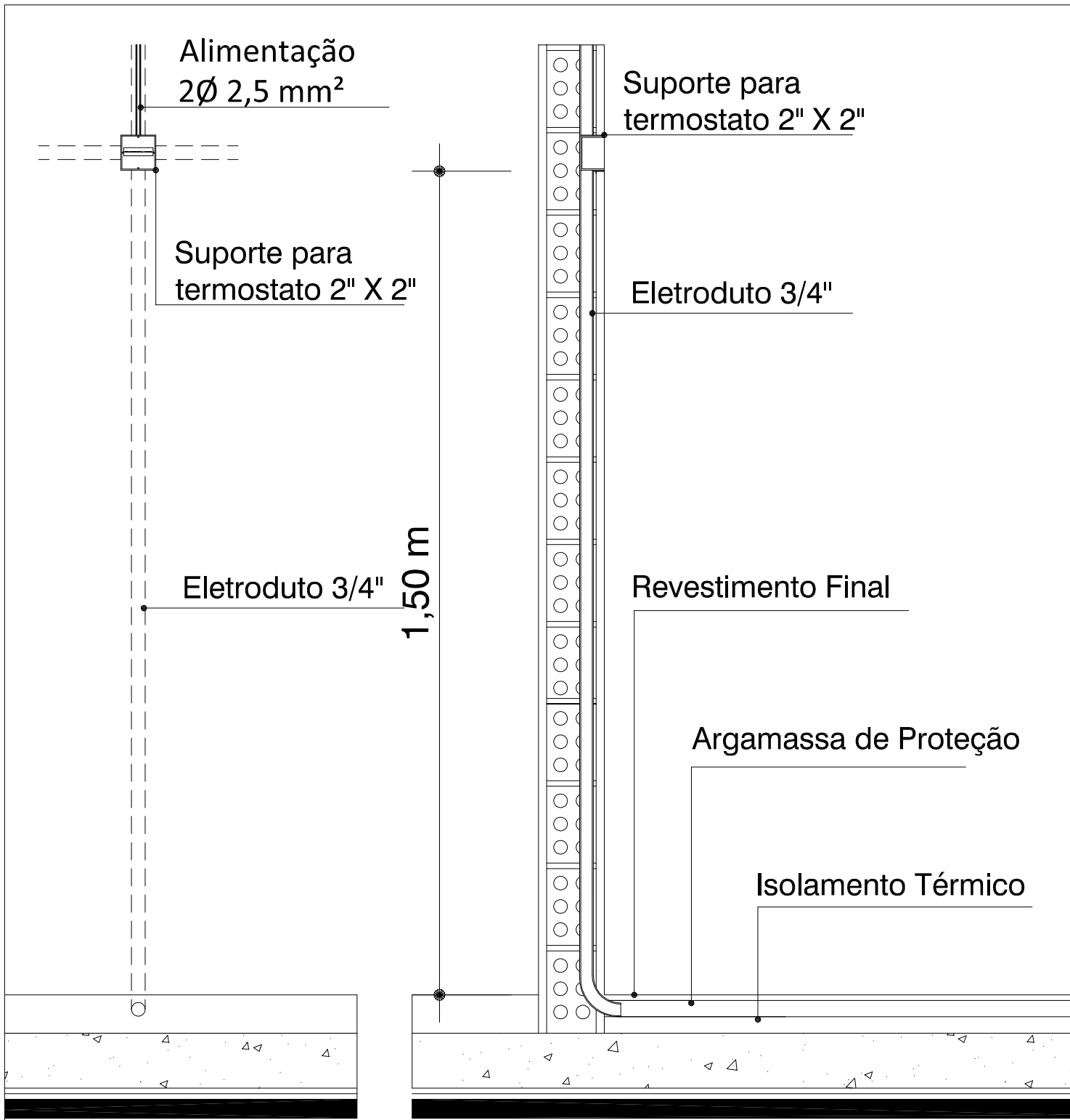
Elevação
